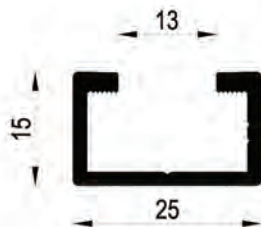
Profilo in alluminio estruso guida 25x15. Lunghezza barre: 6000 mm.
