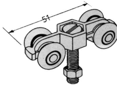
Rodízio 3 Giratório
