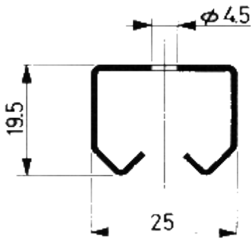
Perfil 180
