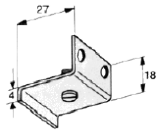
Suporte Lateral 15
