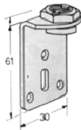
Placa giratória 1107
