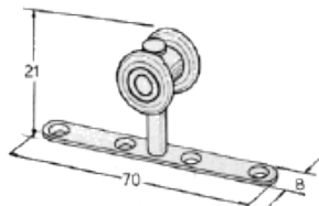
Rodízio 5026
